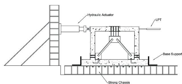
Fig. 5 Test setup
